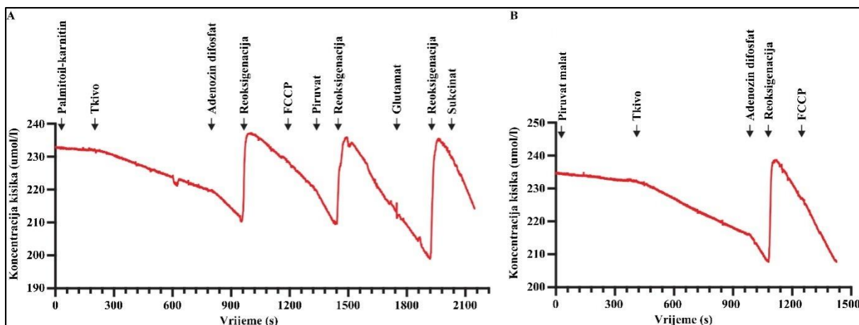
Slika 5. Reprezentativni tragovi iz respirometrijskih mjerenja. Dva eksperimentalna protokola (A i B) su korištena za mjerenje koncentracije kisika prilikom uzastopnog dodavanja supstrata kao što je naznačeno strelicama. Kratice: FCCP – trifluoro karbonilcijanid fenilhidrazon.
